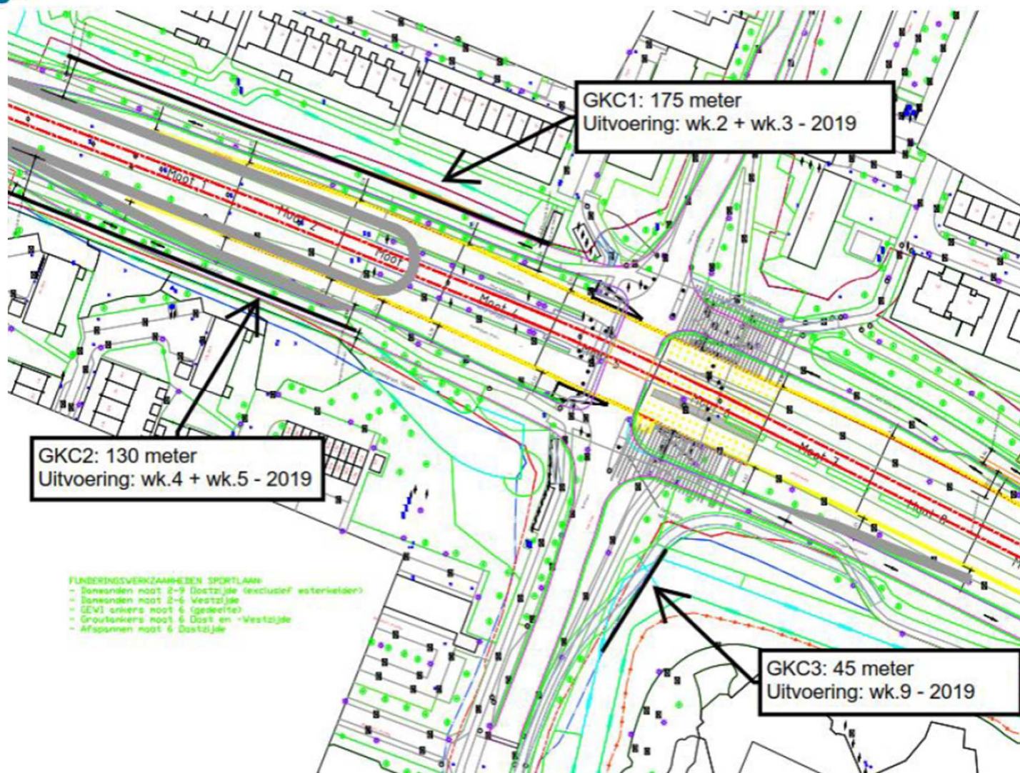
Locaties damwanden
